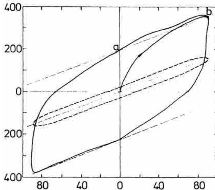
Рис.8. Гистерезисные кривые: сдвигающая сила (кН) – перемещение(мм): для обычной резиноталлической опорной части (пунктирные линии) и для резиноталлической опорной части со свинцовым сердечником (сплошные линии).
