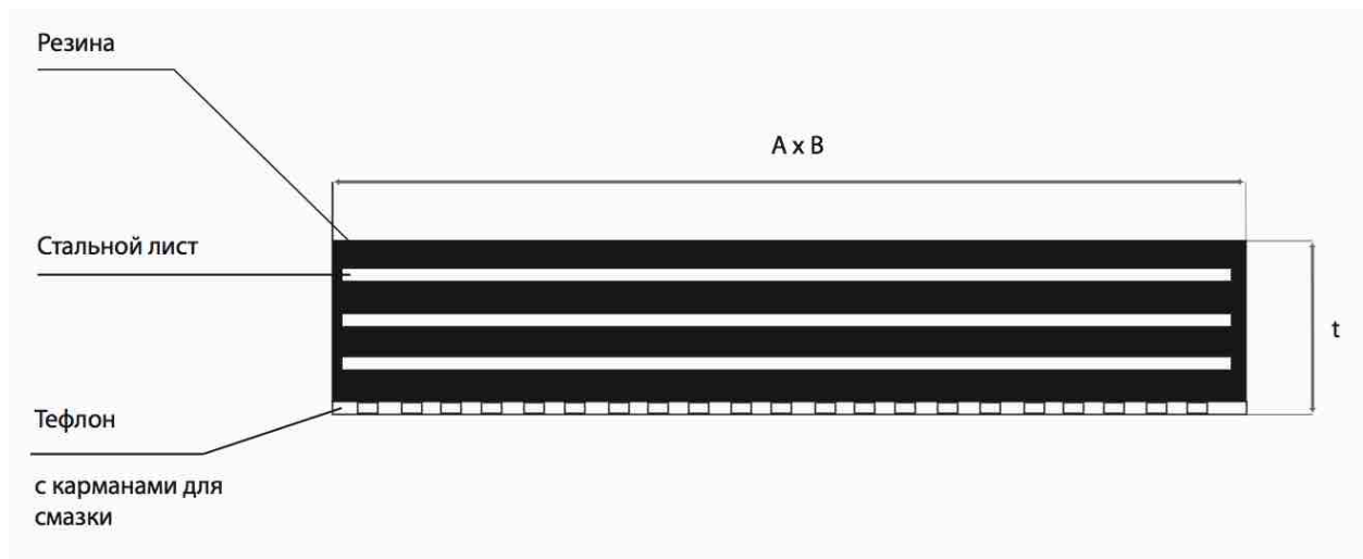
Рисунок 10 – Конструкция карточки скольжения ДШР-КС
