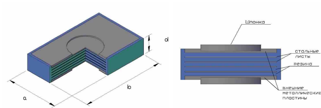
Рисунок А.3 – АШ ДШР-РОЧ. армированная анкеруемая опорная часть с внешними металлическими пластинами и шпонкой.
